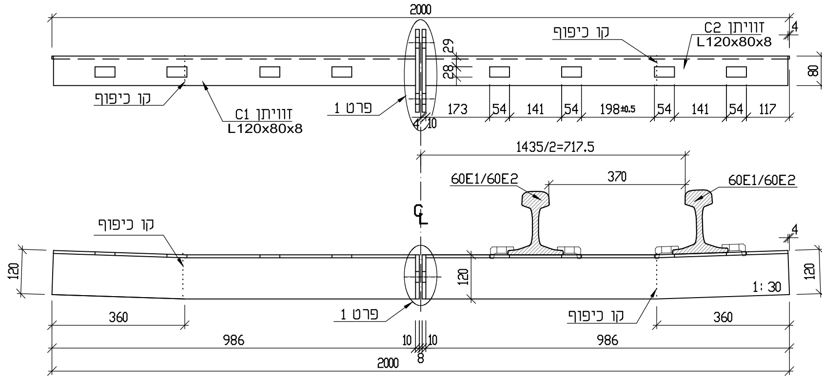
חתך 3-3 - זוויתן מבודד C
