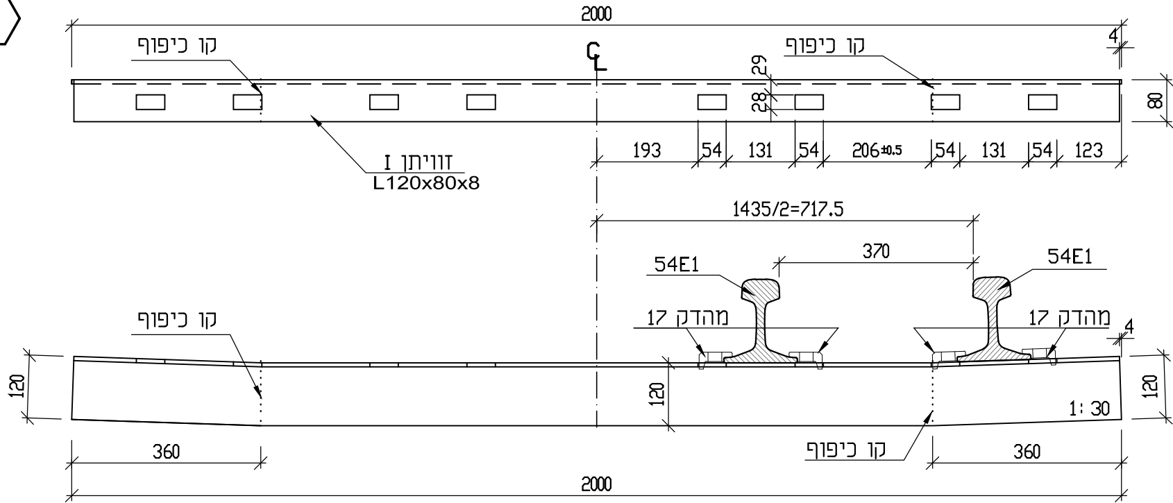
חתך 9-9 - זוויתן I 1:10
